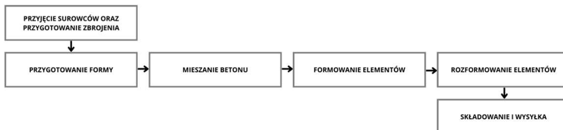
Rysunek 4.1: Uproszczony schemat produkcji elementów żelbetowych
