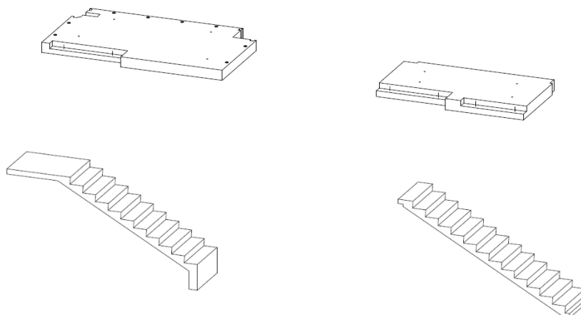
Rysunek 4.2: Elementy schodów
